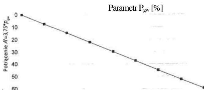
Rys. 1 Graniczne przedstawienie wartości parametru A'
